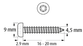
Wkręt montażowy z łbem płasko-soczewkowym z gniazdem TORX 4.5x16 mm lub 4.5x20 mm
